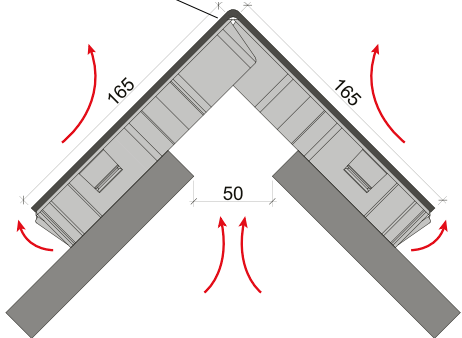
Коньково-карнизная черепица Дёке
